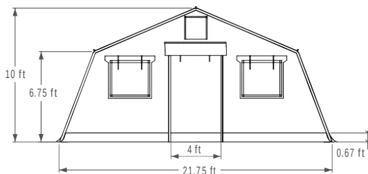
Přední // čelní stěna
