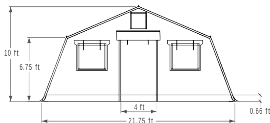
Přední // čelní stěna
