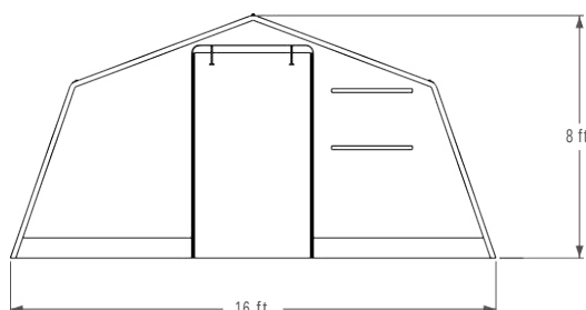
Přední // čelní stěna
